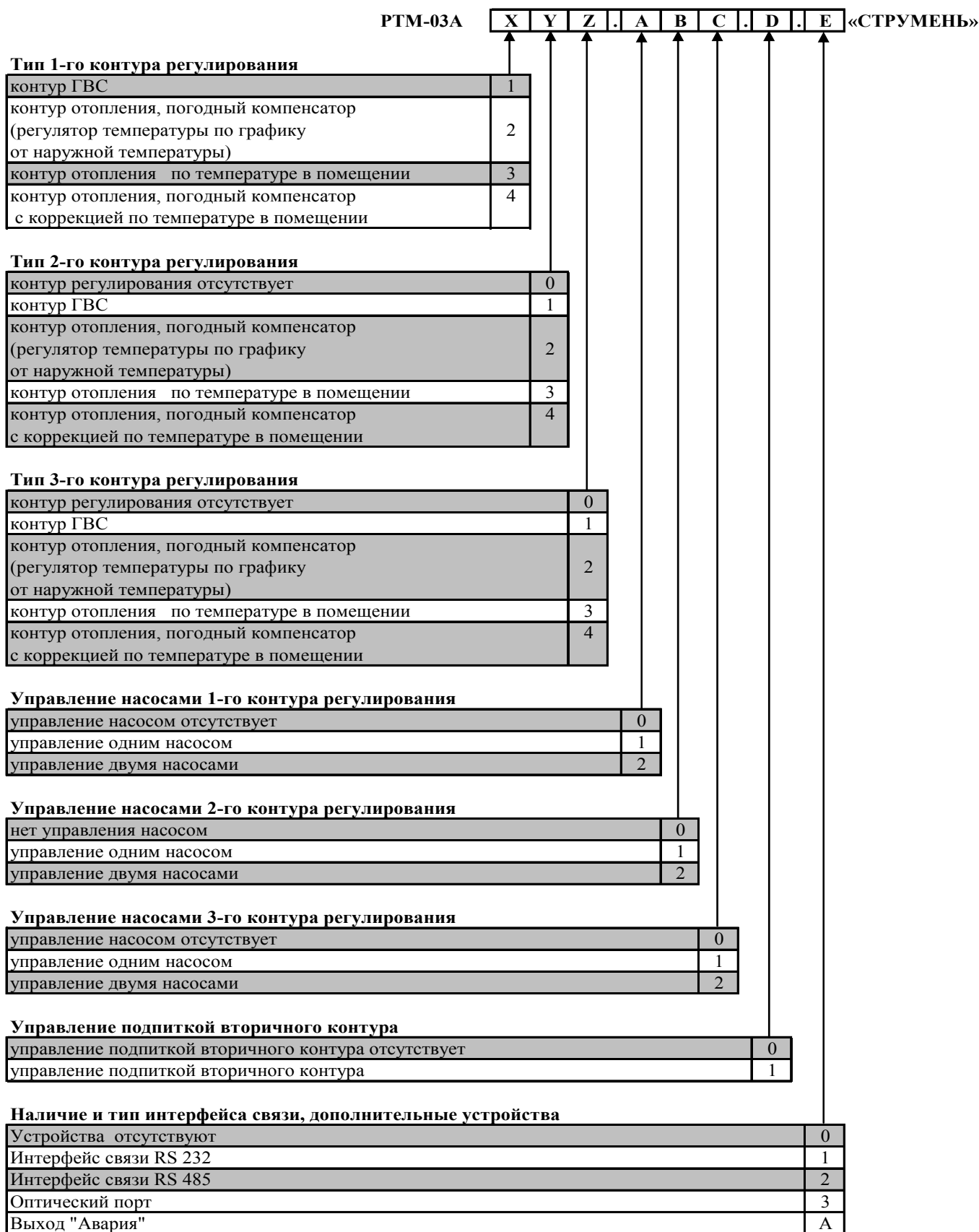
Рисунок 1-Схема обозначений модификаций РТ Пример заказа:
