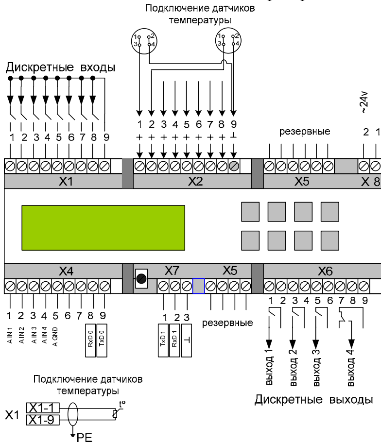
Рисунок А.1- Пример подключения РТ
