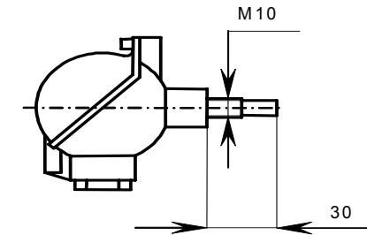
Рис. 6.2. Датчик измерения температуры наружного воздуха (тип ТДВ).
