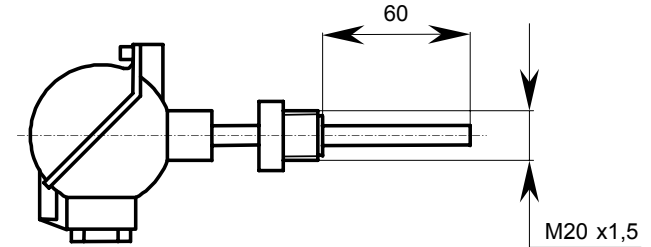
Рис. 6.1. Датчик измерения температуры теплоносителя (тип ТДТ).
