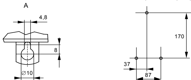
Разметка для крепления прибора
