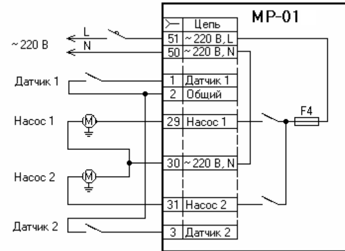
Рис. 4.2 Схема подключения к MP-01 насосов с управлением по датчику перепада давления.
