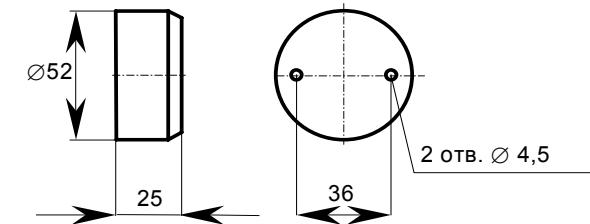
Рис. 6.3. Датчик измерения температуры в помещении (тип ТДП).
